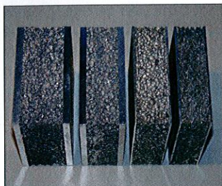
AFS mit verschiedenen Schaum- und Decklagendicken Bild: pohltec metalfoam
